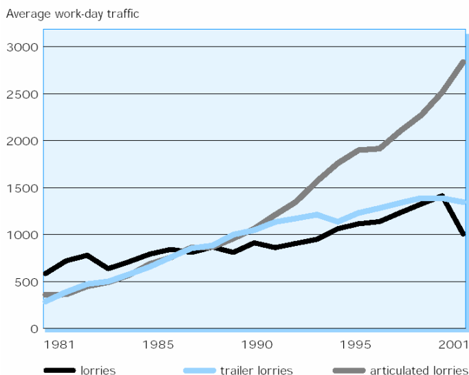
Figuur 7 Evolutie van het aantal vrachtwagens dat door de Zwitserse Alpen rijdt
